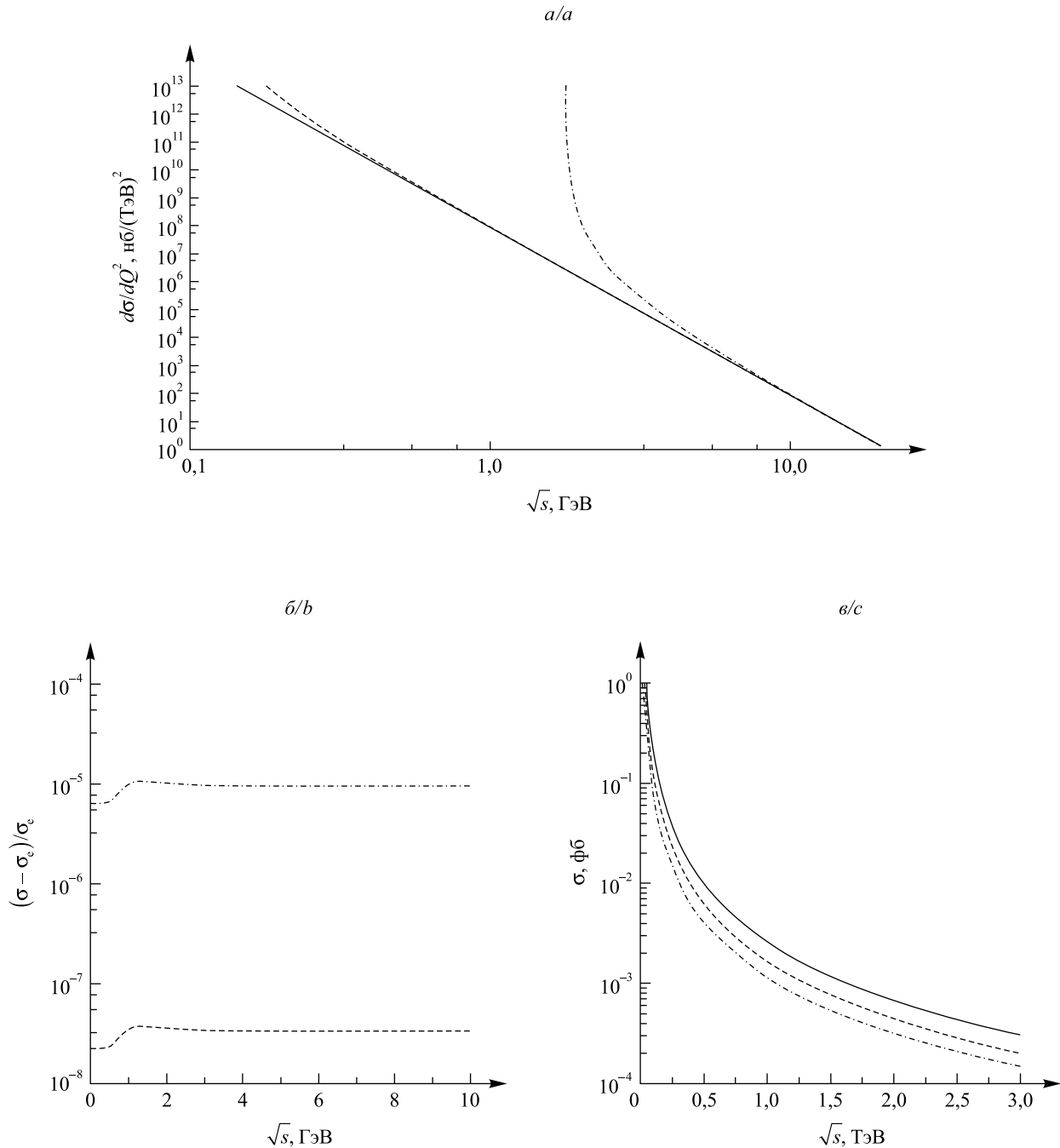
Рис. 4. Сечения рассеяния d\sigma/dQ^2 (а), (\sigma - \sigma_e)/\sigma_e (б), \sigma (в) фотонов на различных типах лептонов:
