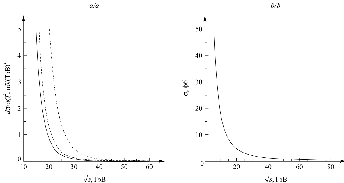
Рис. 2. Сечения рассеяния d\sigma/dQ^2 (а), \sigma (б) при следующих значениях \sqrt{Q^2} : ——— 800 МэВ; - - - - - 1 ТэВ; ······ 3 ТэВ Fig. 2. Scattering cross sections d\sigma/dQ^2 (а), \sigma (б) for the following values of \sqrt{Q^2} : ——— 800 MeV; - - - - - 1 TeV; ······ 3 TeV
