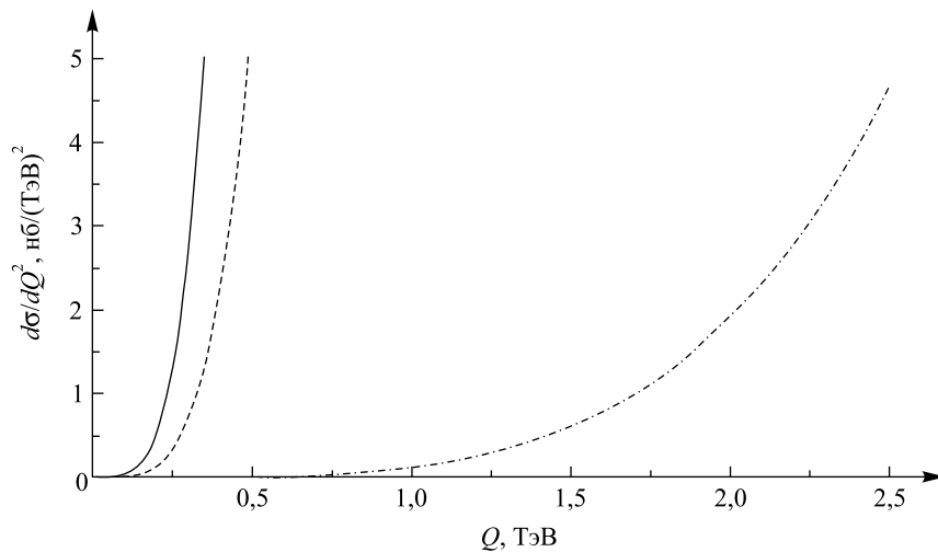
Рис. 3. Сечение рассеяния d\sigma/dQ^2 при следующих значениях энергии взаимодействия: ————— 800 МэВ; - - - - - 1 ТэВ; - · - · - 3 ТэВ Fig. 3. Scattering cross sections d\sigma/dQ^2 for the following values of the interaction energy: ————— 800 MeV; - - - - - 1 TeV; - · - · - 3 TeV
