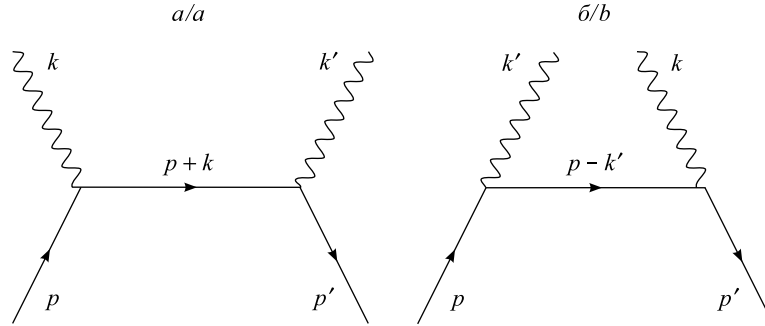
Рис. 1. Диаграммы процесса l\gamma \rightarrow l\gamma в борновском приближении: а – исходная диаграмма; б – кроссинг-симметричная диаграмма Fig. 1. Diagrams of l\gamma \rightarrow l\gamma process in the Born approximation: а – original diagram; б – crossing symmetric diagram
