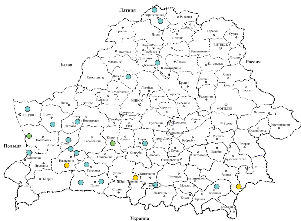
Рис. 2. Карта локализации гаплотипов дуба черешчатого (продолжение): в – гаплотип № 3 и его производные; з – гаплотип № 7 и его производные
