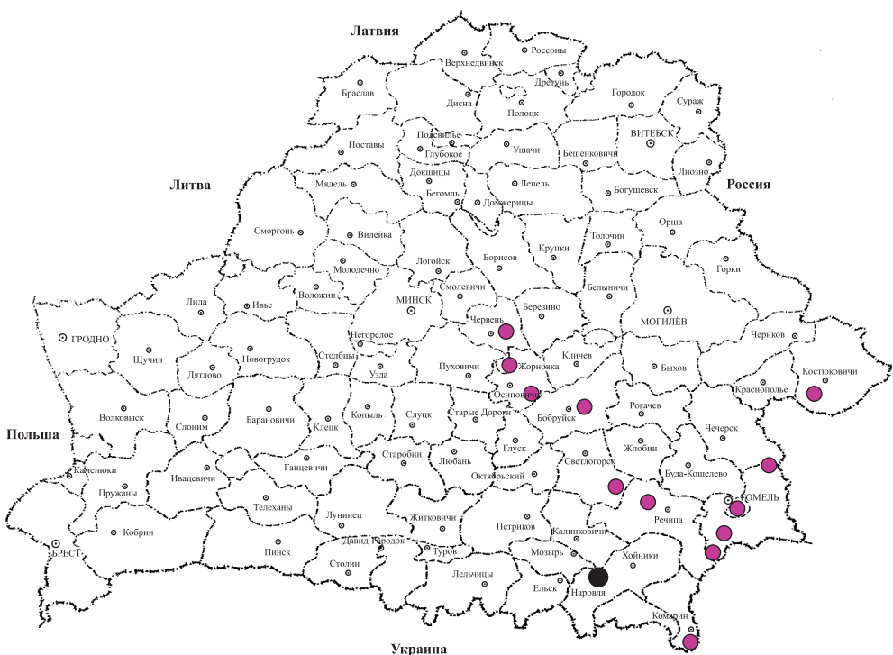
Рис. 2. Карта локализации гаплотипов дуба черешчатого (начало): а – гаплотип № 1 и его производные; б – гаплотип № 2 и его производные
