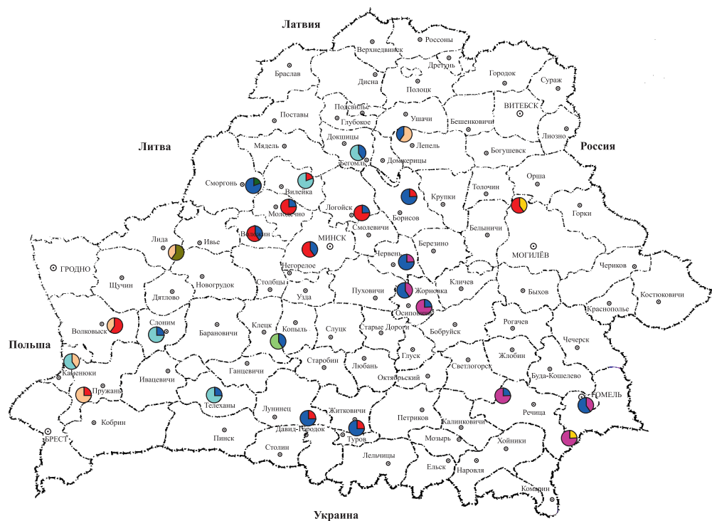
Рис. 2. Карта локализации гаплотипов дуба черешчатого (окончание):
