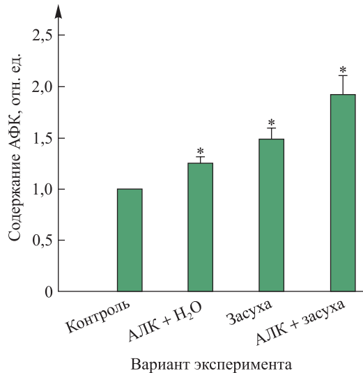
Рис. 2. Изменение содержания АФК в листьях растений ячменя сортов Бровар ( а ) и Аванс ( б ), обработанных АЛК, под воздействием почвенной засухи (звездочкой отмечены достоверные различия по сравнению с контролем ( p \leq 0,05 ))
