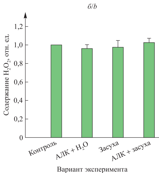
Рис. 3. Изменение содержания H_2O_2 в листьях растений ячменя сортов Бровар ( а ) и Аванс ( б ), обработанных АЛК, под воздействием почвенной засухи
