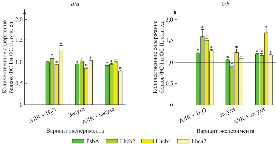
Рис. 6. Содержание белков ФС I и ФС II в листьях растений ячменя сортов Бровар ( a ) и Аванс ( б ), обработанных АЛК, в условиях почвенной засухи (контроль принят за единицу и представлен базовой линией; звездочкой отмечены достоверные различия по сравнению с контролем ( p \leq 0,05 ))
