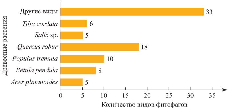
Рис. 3. Количество видов фитофагов, трофически связанных с отдельными видами древесных растений на территории республиканского ландшафтного заказника «Озеры»
