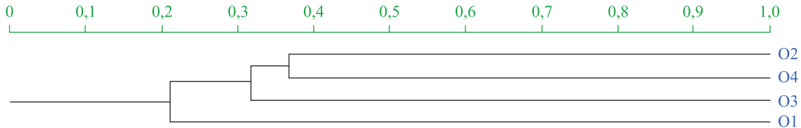
Рис. 4. Дендрограмма сходства сообществ фитофагов по видовому составу (индекс Чекановского – Сёренсена) на исследованных пробных площадях республиканского ландшафтного заказника «Озеры»
