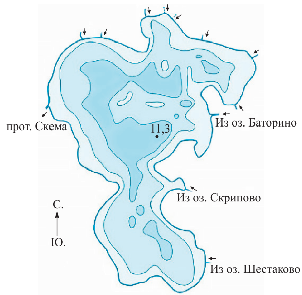
Рис. 3. Карта и батиметрическая схема оз. Мястро.
