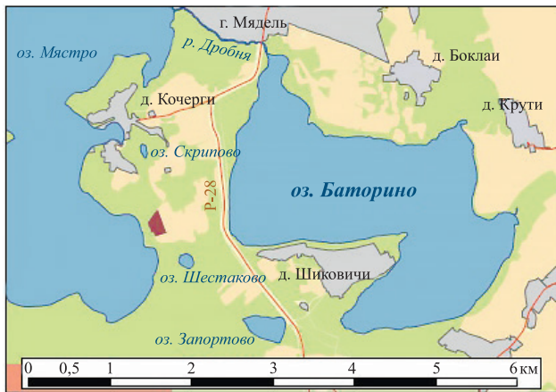
Рис. 4. Карта и батиметрическая схема оз. Баторино.
