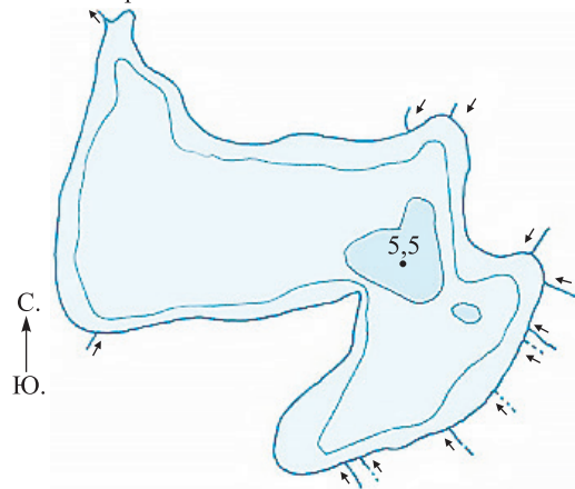
Рис. 4. Карта и батиметрическая схема оз. Баторино.
