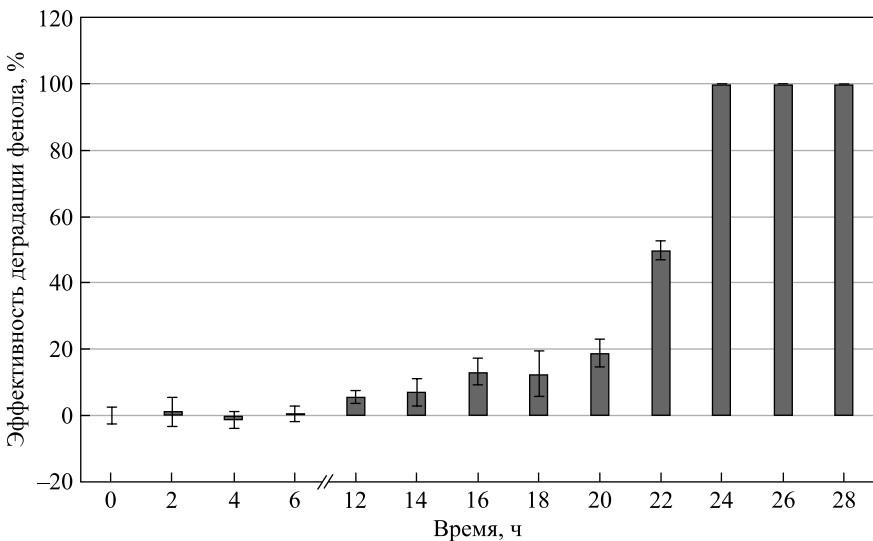
Рис. 3. Эффективность деградации фенола (200 мг/л) бактериями штамма R. pyridinivorans 5Ap.
