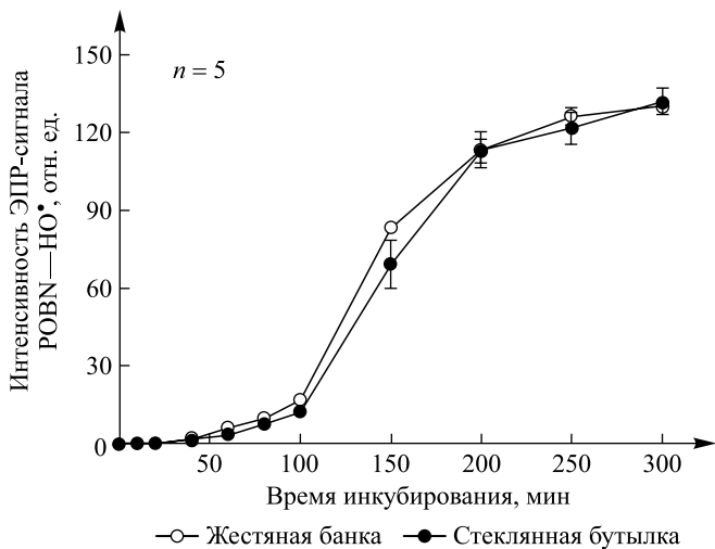
Рис. 3. Изменение интенсивности ЭПР-сигнала спинового аддукта \text{POBN—HO}^\bullet в образце пива сорта «Золото пивовара» в зависимости от времени инкубирования
