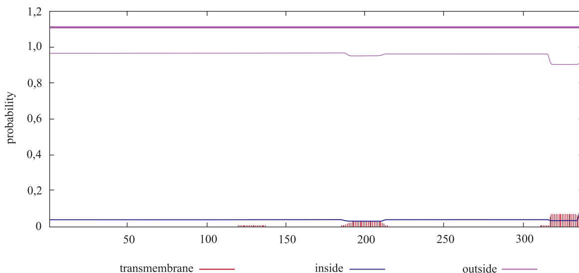
Рис. 5. Результат анализа локализации изучаемого белка
