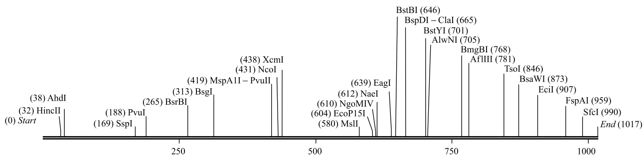
Рис. 1. Рестрикционная карта acdS -гена бактерий P. putida B-37, построенная с помощью программы SnapGene ( http://www.snapgene.com/ )
