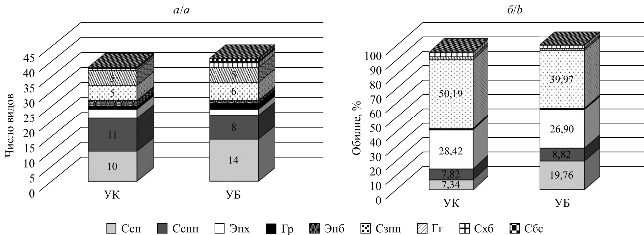
Рис. 2. Соотношение групп жизненных форм жуужелиц по числу видов (а) и относительному обилию (б) в биоценозах (УК – без борщевика, УБ – с засорением борщевиком)
