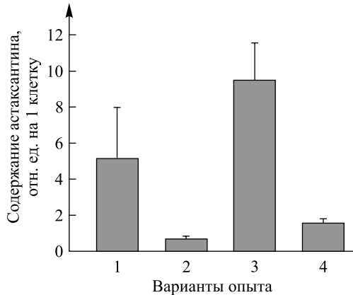
Рис. 2. Количество астаксантина в клетках H. pluvialis через 21 сут эксперимента на полной среде Рудика (варианты 1, 3) и среде Рудика без азота (варианты 2, 4), при освещенности 1500 лк (варианты 1, 2) и 10 000 лк (варианты 3, 4)
