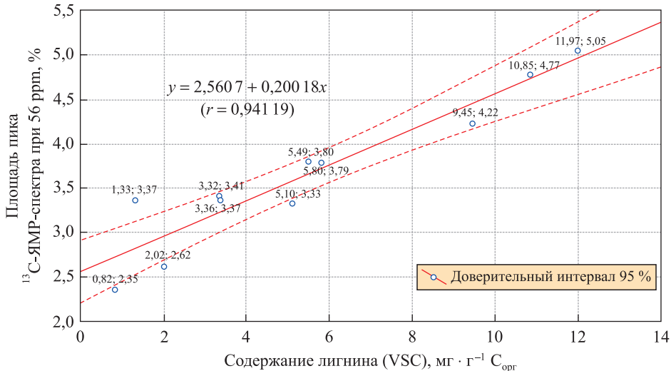
Рис. 6. Коэффициент корреляции между содержанием лигнина (VSC) и площадью пика ^{13}\text{C} -ЯМР-спектра при 56 ppm
