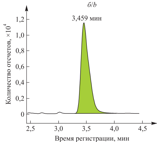
Рис. 2. Внутриклеточное содержание пролина в клетках штамма P. megaterium Cp-1: a – без хлорида натрия (контроль); б – в присутствии 1197 ммоль/л NaCl
