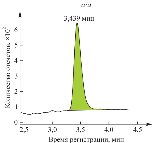
Рис. 2. Внутриклеточное содержание пролина в клетках штамма P. megaterium Cp-1: a – без хлорида натрия (контроль); б – в присутствии 1197 ммоль/л NaCl
