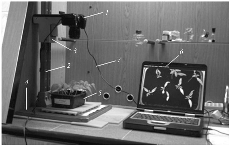
Рис. 1. Установка для метода DISP: 1 – фотокамера; 2 – стойка штатива; 3 – регулируемый по высоте держатель фотокамеры; 4 – основание штатива; 5 – контейнер с проростками;
