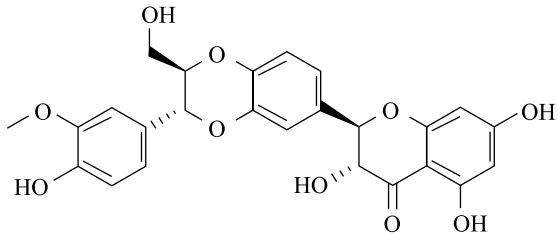
Рис. 1. Структурные формулы исследованных соединений: a – силибин; б – акацетин
