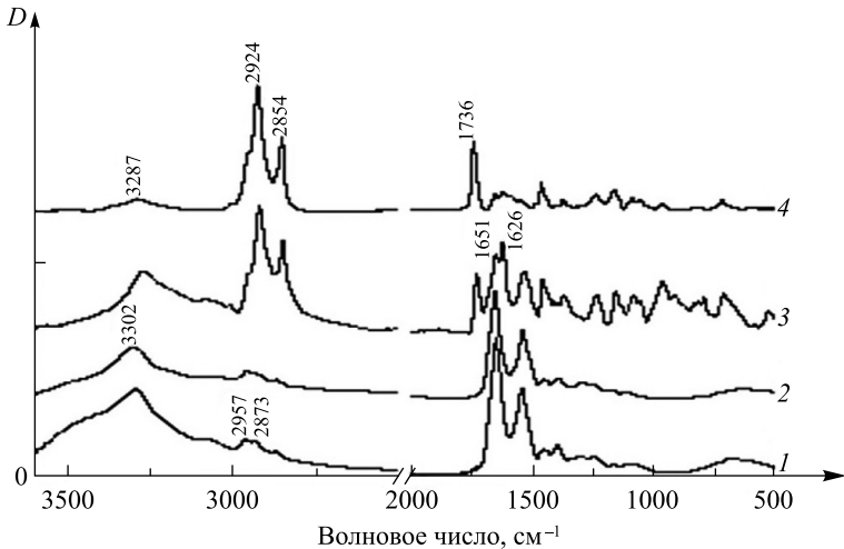
Рис. 2. ИК фурье-спектры пленок плазмы крови контрольной группы (1), альбумина (2), ЛПНП (3) и ЛПОНП (4) в области частот 3600–500 см -1 (для наглядности спектры смещены по оси ординат)
