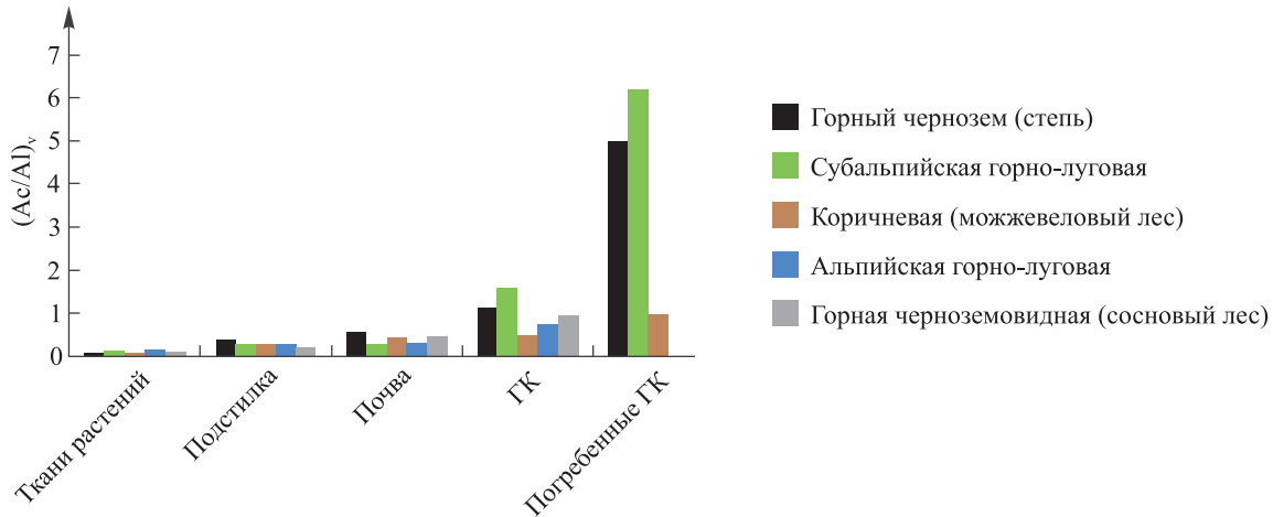
Рис. 4. Величины отношения ванилиновых кислот к ванилину ((Ac/Al)_v) на разных стадиях трансформации лигнина в ряду растительные ткани – опад – подстилки – почвы – гуминовые кислоты (ГК) – погребенные гуминовые кислоты
