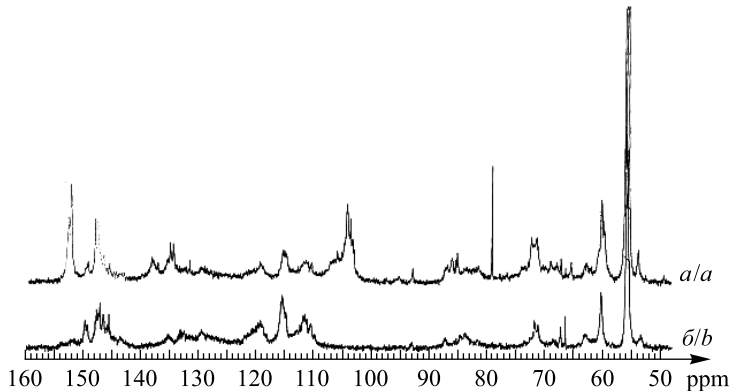
Рис. 9. ^{13}\text{C} -ЯМР-спектры нативных препаратов лигнина древесных культур: а – акация; б – лиственница. Источник: [14]
