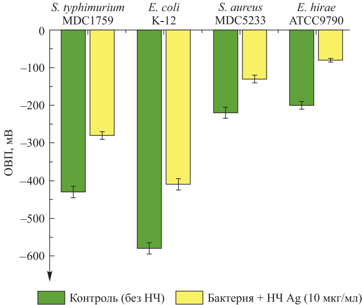
Рис. 4. Изменение ОВП среды различных бактерий при росте в присутствии НЧ Ag (10 мкг/мл). Контроль – бактерии, выращенные без НЧ
