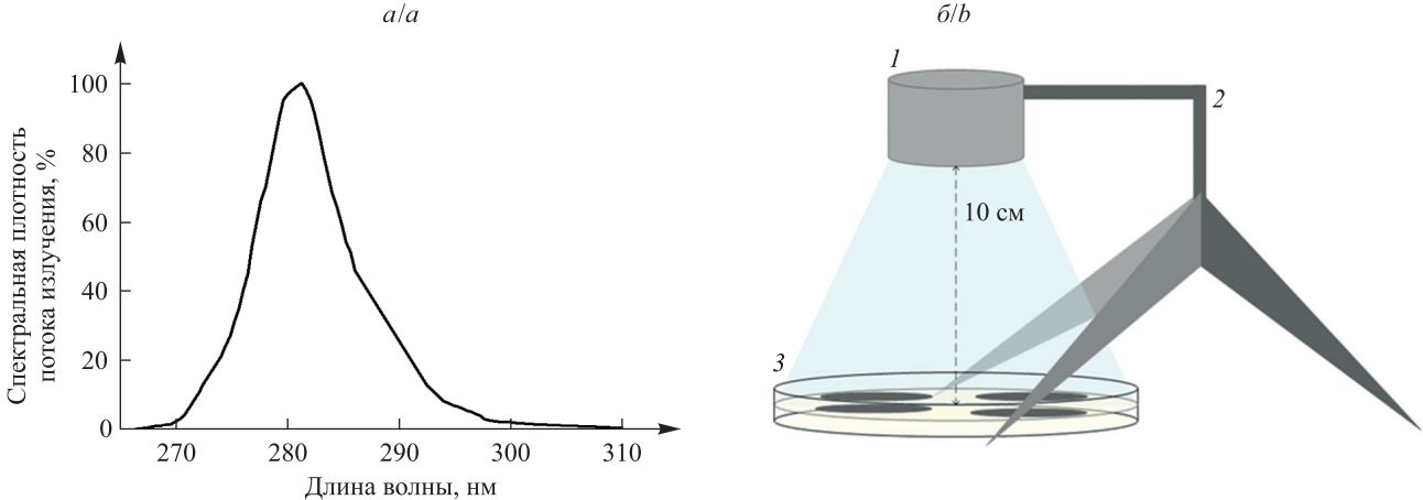
Рис. 1. Спектр излучения диодного источника УФ-С ( а ) и схема установки для облучения колоний грибов ( б ): 1 – УФ-диод; 2 – штатив; 3 – чашка Петри с колониями микромицетов
