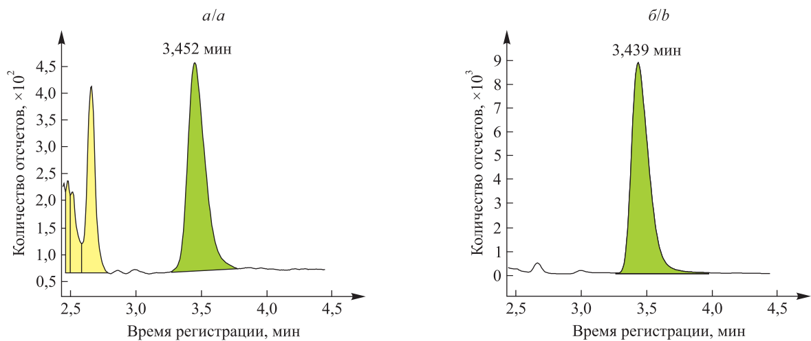
Рис. 3. Внутриклеточное содержание пролина в клетках штамма Rh. jostii CA-6: a – без хлорида натрия (контроль); б – в присутствии 1197 ммоль/л NaCl
