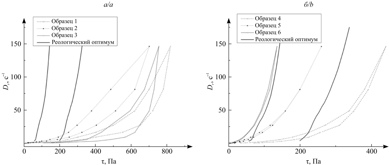
Рис. 1. Влияние концентрации пластификаторов и гелеобразователя на реологические свойства гелей МЦ при 20 °С: a – образцы 1–3; б – образцы 4–6
