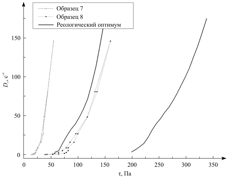
Рис. 3. Реограмма течения гелей карбопола при 20 °С
