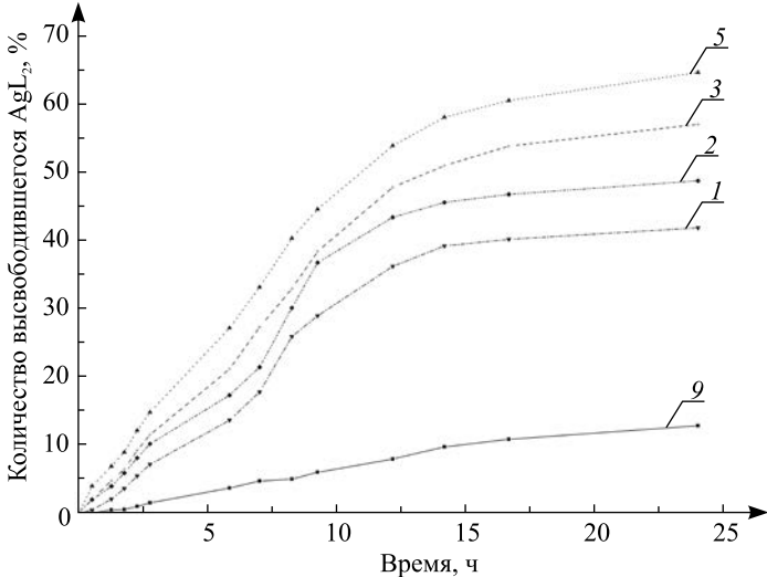
Рис. 4. Кинетический профиль высвобождения комплекса \text{AgL}_2 из образцов мазей (номер образца указан на кривой)
