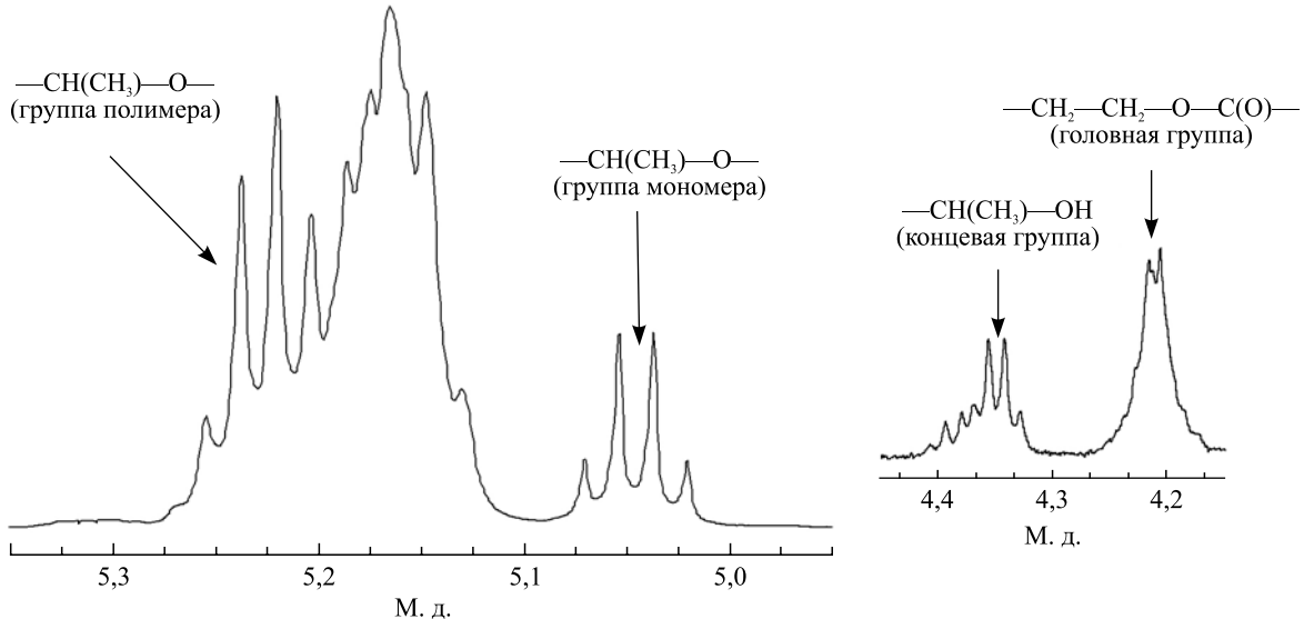
Рис. 1. Фрагменты спектра ЯМР ^1\text{H} поли(D,L-Ла)
