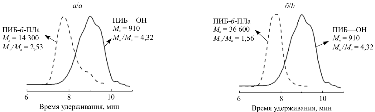
Рис. 6. Кривые ГПХ образцов поли(ИБ-блок-D,L-Ла) для [D,L-Ла] : [ПИБ—ОН], равного 100 ( a ) и 200 ( б ) Fig. 6. GPC curves for poly(isobutylene- b -D,L-lactide) for [D,L-lactide] : [PIB—OH] equal to 100 ( a ) and 200 ( b )
