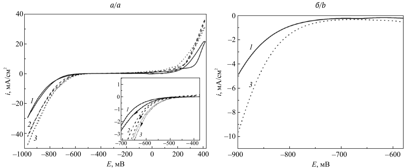
Рис. 1. Фоновый электролит (без \text{Sn(II)} и \text{Ag(I)} ): а – ЦВА-кривые для медного рабочего электрода с покрытием Ni-P; б – катодные сканы ЦВА-кривых для рабочего электрода – оловянной фольги. Температура электролита, °C: 1 – 20; 2 – 40; 3 – 60
