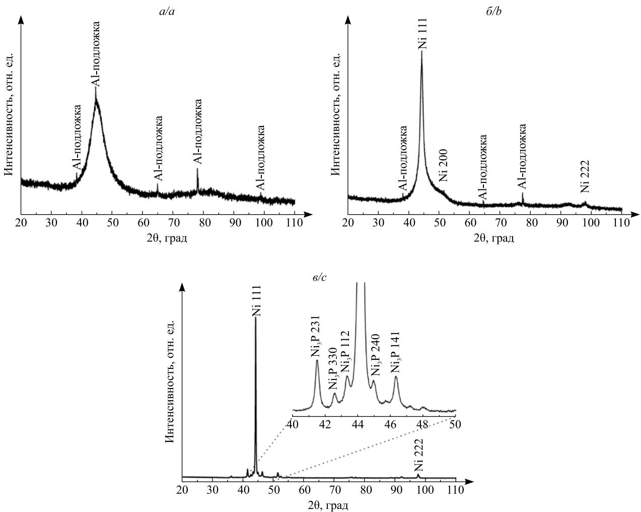
Рис. 2. Рентгеновские дифрактограммы от свежесажженного покрытия Ni-P (а) и покрытий, нагретых до 250 °C (б), 400 °C (в)
