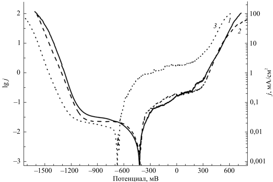
Рис. 3. Анодные и катодные поляризационные кривые, записанные для покрытий Ni–P до отжига (1) и покрытий, отожженных при 250 °C (2) и 400 °C (3)
