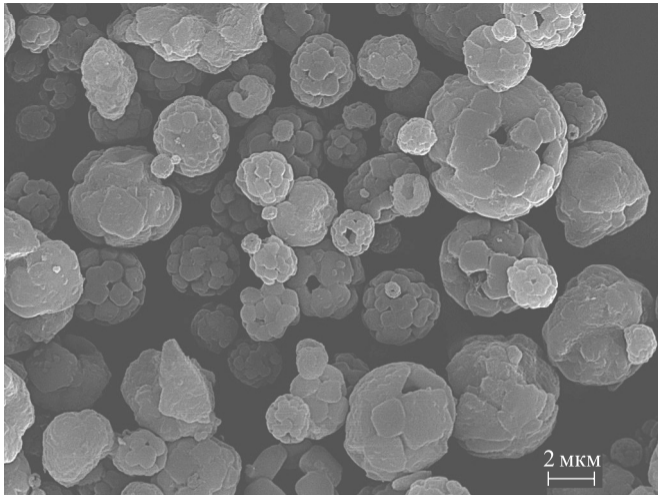
Рис. 1. СЭМ-изображение продукта распылительной сушки суспензии наночастиц \text{Mg}_{0,5}\text{Zn}_{0,5}\text{Fe}_2\text{O}_4 в присутствии NaCl Fig. 1. SEM image of \text{Mg}_{0,5}\text{Zn}_{0,5}\text{Fe}_2\text{O}_4 nanoparticle suspension spray-dried in presence of NaCl
