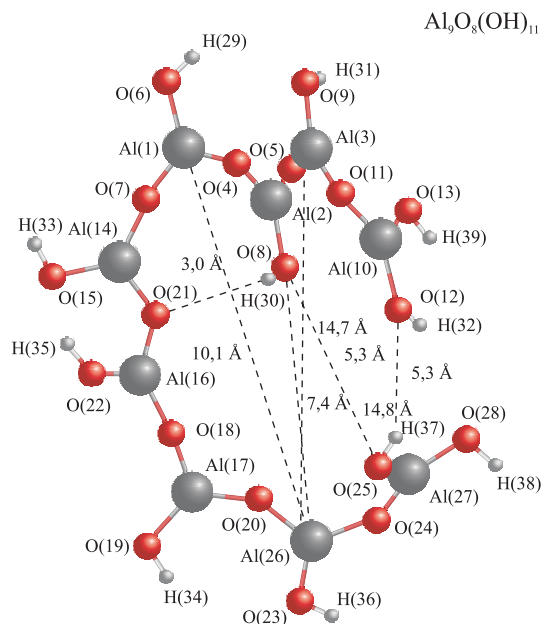
Рис. 4. Структуры моно- и полиядерных гидроксокомплексов алюминия
