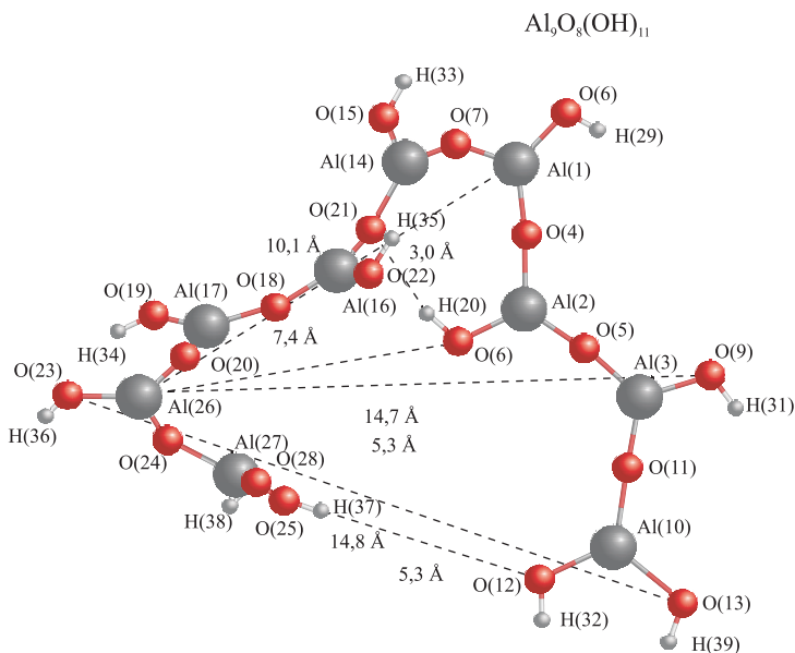
Рис. 4. Структуры моно- и полиядерных гидроксокомплексов алюминия
