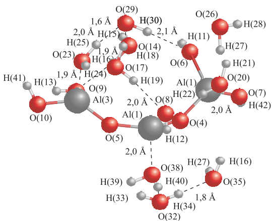
Рис. 5. Структуры гидратированных моно- и полиядерных гидроксокомплексов алюминия
