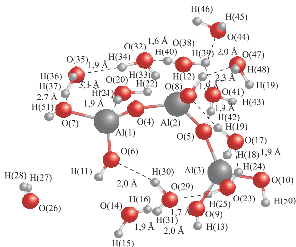
Рис. 5. Структуры гидратированных моно- и полиядерных гидроксокомплексов алюминия
