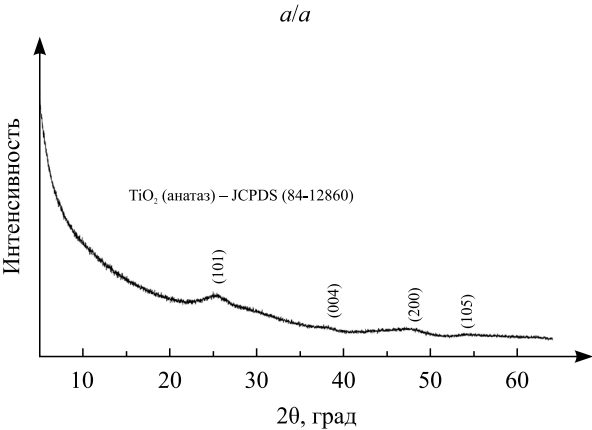
Рис. 4. Рентгеновская дифрактограмма ( a ) и ИК-спектр ( b ) \text{TiO}_2 , полученного гидролитическим синтезом из \text{Na}_2\text{Ti}_3\text{O}_7
