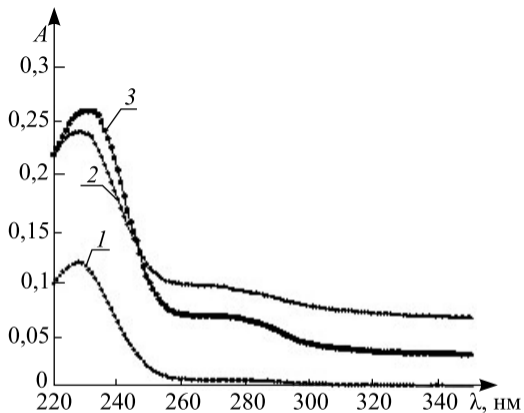
Рис. 2. УФ-спектры ГЭ n -ТФАБК (система 1 из табл. 1):
