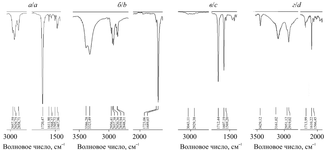
Рис. 7. ИК-спектры: a – ГЭ n -ТФАБК; б – гидратной формы ГЭ n -ТФАБК; в – n -МТФАФ; г – гидратной формы n -МТФАФ
