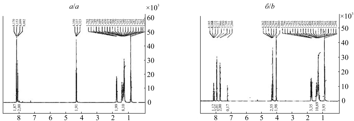
Рис. 8. Спектры ЯМР ^1\text{H} : a – ГЭ n -ТФАБК; б – гидратной формы ГЭ n -ТФАБК
