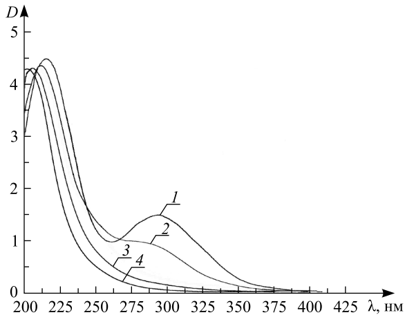
Рис. 6. Оптические спектры 5 \cdot 10^{-4} моль/л раствора \text{H[AuCl}_4\text{]} при значениях pH: 1 – 3,0; 2 – 4,5; 3 – 6,0; 4 – 12,0 Fig. 6. Optical spectra of 5 \cdot 10^{-4} mol/L \text{H[AuCl}_4\text{]} solution at different pH values: 1 – 3.0; 2 – 4.5; 3 – 6.0; 4 – 12.0
