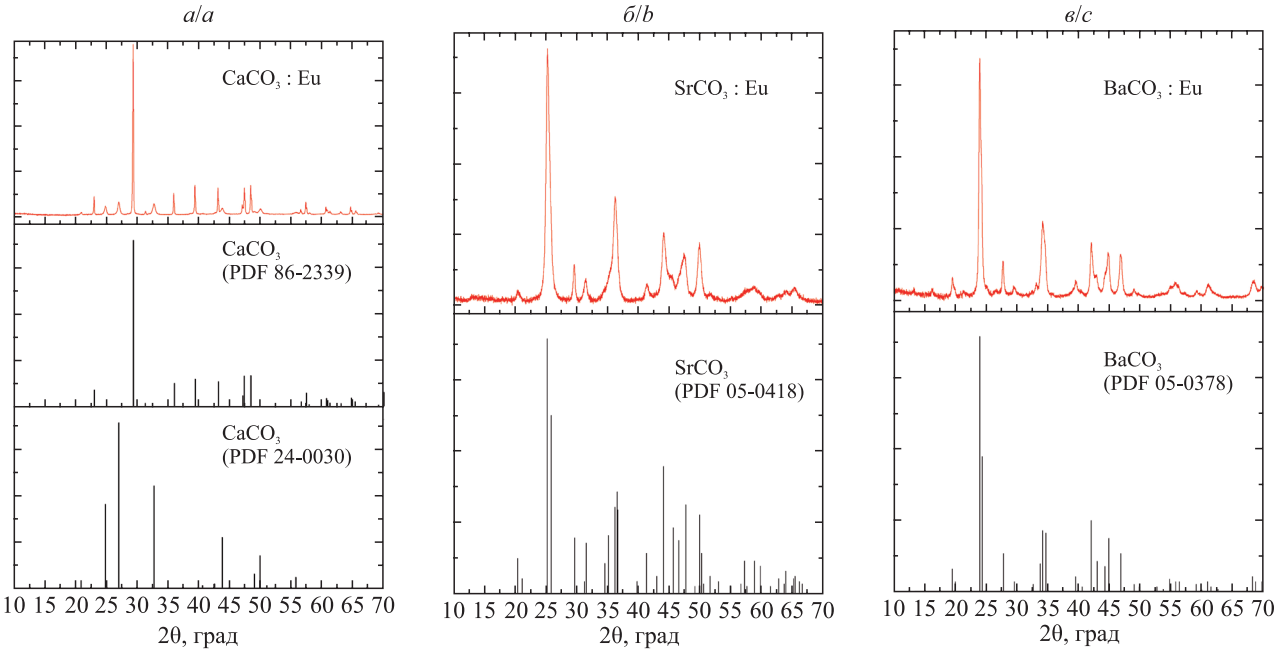
Рис. 1. Рентгенограммы образцов: a - \text{CaCO}_3:\text{Eu}^{3+} ; \delta - \text{SrCO}_3:\text{Eu}^{3+} ; \epsilon - \text{BaCO}_3:\text{Eu}^{3+}
