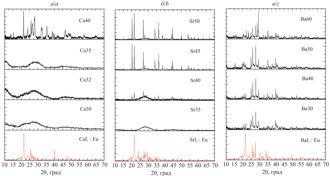
Рис. 4. Рентгенограммы образцов стеклокерамики на основе \text{CaI}_2 : \text{Eu}^{2+} (а), \text{SrI}_2 : \text{Eu}^{2+} (б), \text{BaI}_2 : \text{Eu}^{2+} (в). Обозначения соответствуют табл. 1
