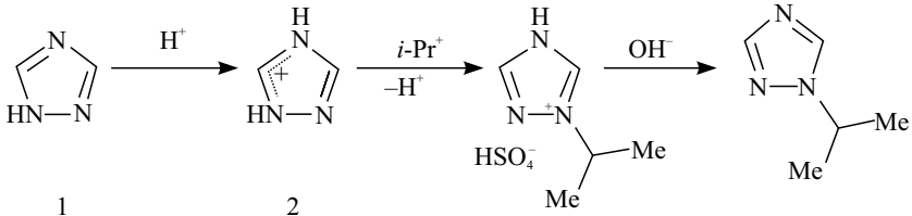
Рис. 2. Схема образования 1-изо-пропил-1H-1,2,4-триазола Fig. 2. Scheme for the formation of 1-iso-propyl-1H-1,2,4-triazole
