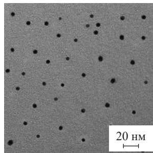
Рис. 2. ПЭМ-изображения наночастиц диоксида титана в ксерогеле, полученном из золя \text{TiO}_2 ( а, б ) и наночастиц золота ( в )
