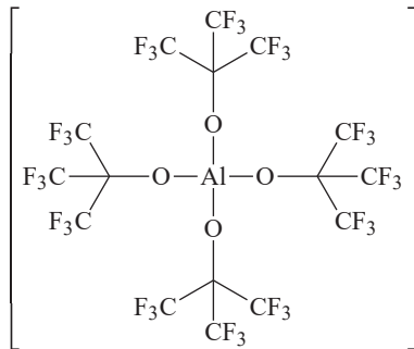
Рис. 3. Каталитические системы, представляющие собой комплексы металлов с нитрильными лигандами, ассоциированные со слабонуклеофильными противоионами
