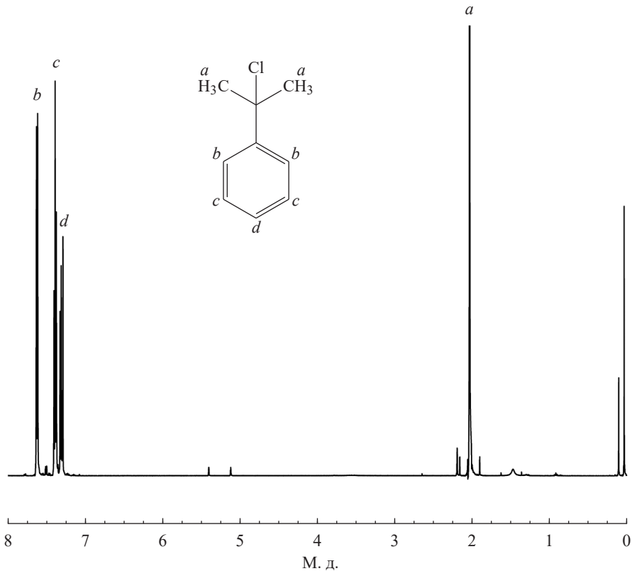
Рис. 1. Спектр ЯМР ^1\text{H} синтезированного кумилхлорида
