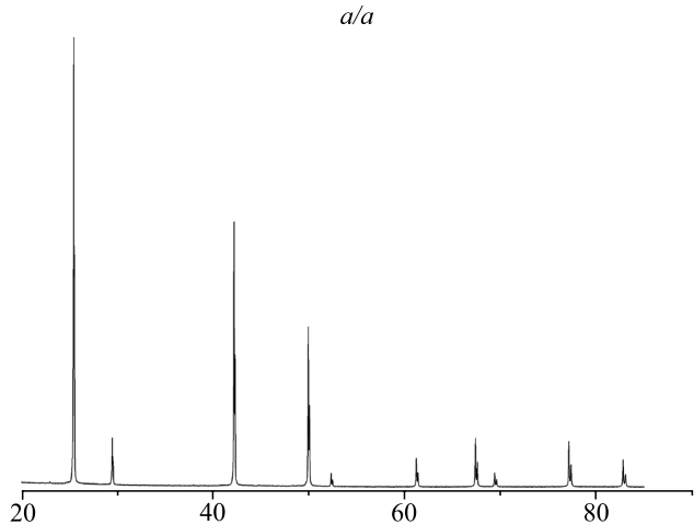
Рис. 1. Рентгенограмма (а) и СЭМ-изображение (б) порошка CuI Fig. 1. XRD patterns (a) and SEM-image (b) for CuI powder
