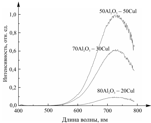
Рис. 3. СЛ (а) и СВЛ (б) однослойных пленок \text{Al}_2\text{O}_3 - \text{CuI} в зависимости от соотношения компонентов (мас. %)
