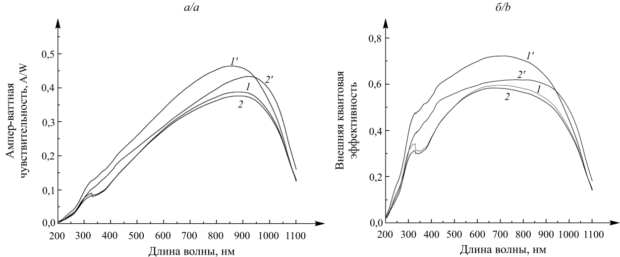
Рис. 5. Спектры ампер-ваттной фоточувствительности ( а ) и внешней квантовой эффективности ( б ) исходных СЭ-1 ( 1 ), СЭ-2 ( 2 ) и СЭ с пленкой состава 50\text{Al}_2\text{O}_3 - 50\text{CuI} (1 слой ( 1' ) и 2 слоя ( 2' ))
