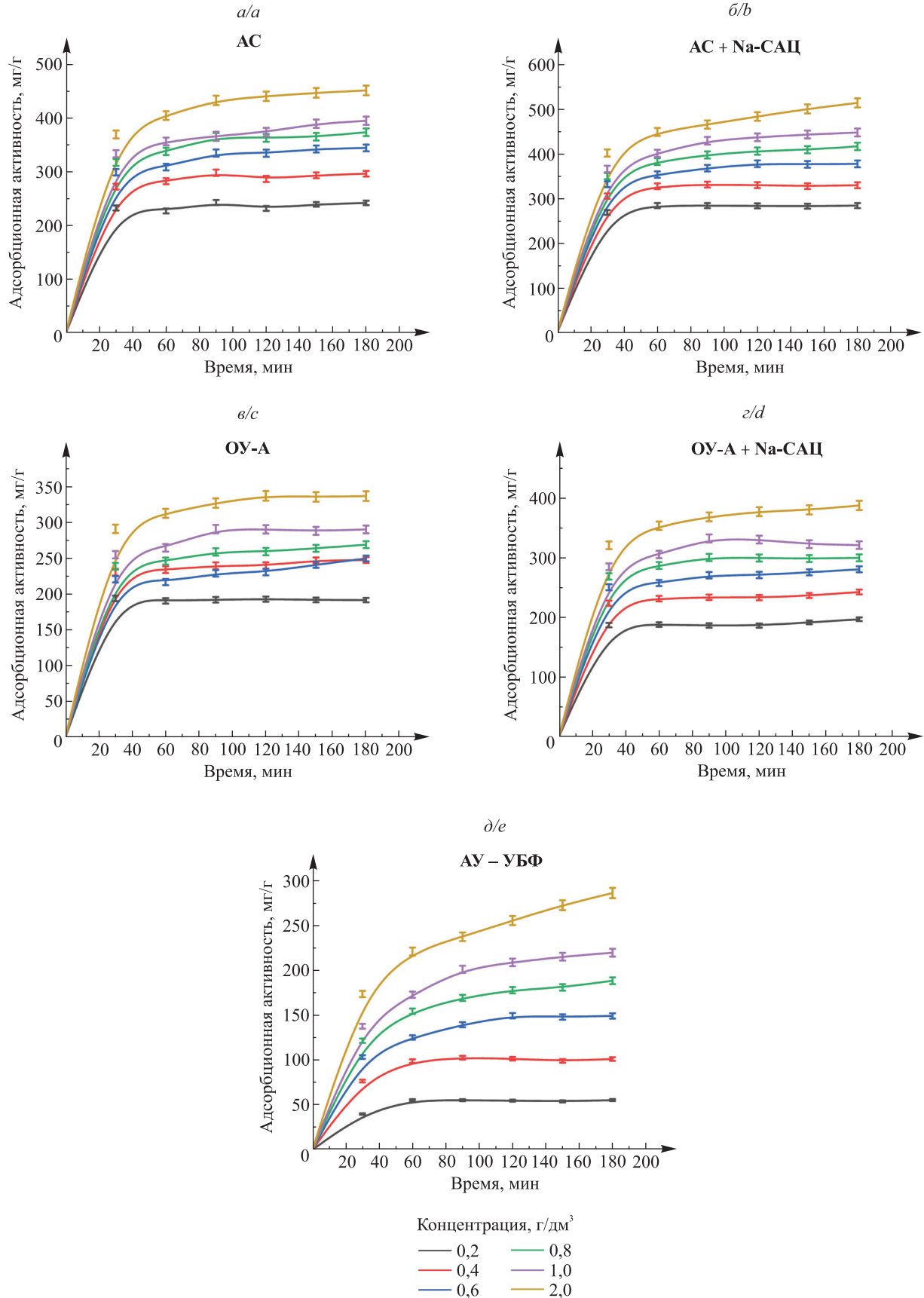
Рис. 1. Кинетические кривые адсорбции МГ угольными энтеросорбентами (а – д)
